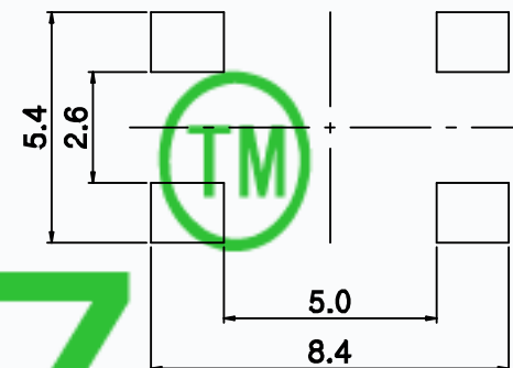
P.C.B. LAND PATTERN
