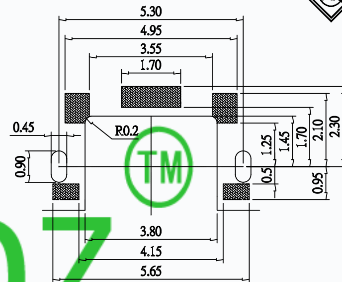
P.C.B. LAND PATTERN
