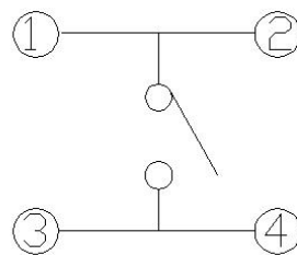
电器原理图
