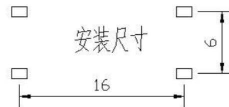
P.C.B. LAND PATTERN
