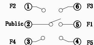
电 路 图
