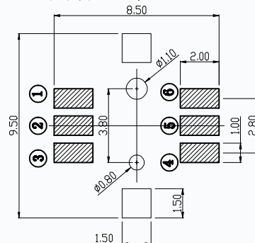
印制板安装孔图
