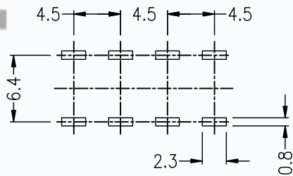
P.C.BOARD LAYOUT
