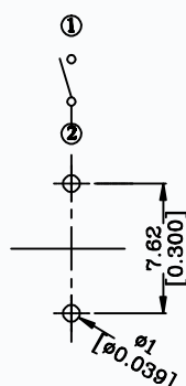
P.C.B LAYOUT
